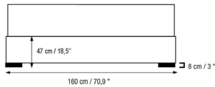
VUE DE FACE / FRONT VIEW
